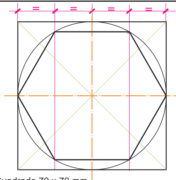
Cuadrado 70 x 70 mm
