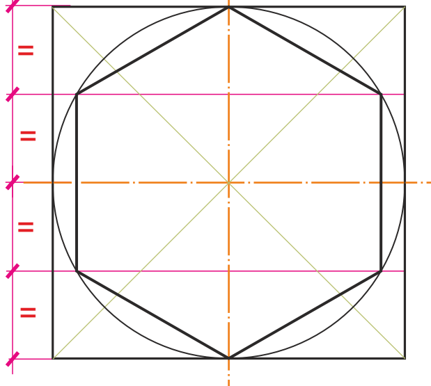
Cuadrado 70 x 70 mm
