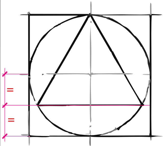
EQUILÁTERO INSCRITO EN CIRCUNFERENCIA 1
