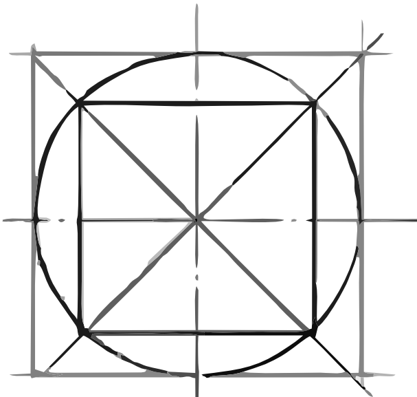
CUADRADO INSCRITO EN CIRCUNFERENCIA 2
