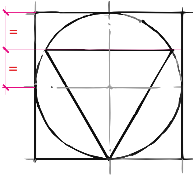
EQUILÁTERO INSCRITO EN CIRCUNFERENCIA 2
