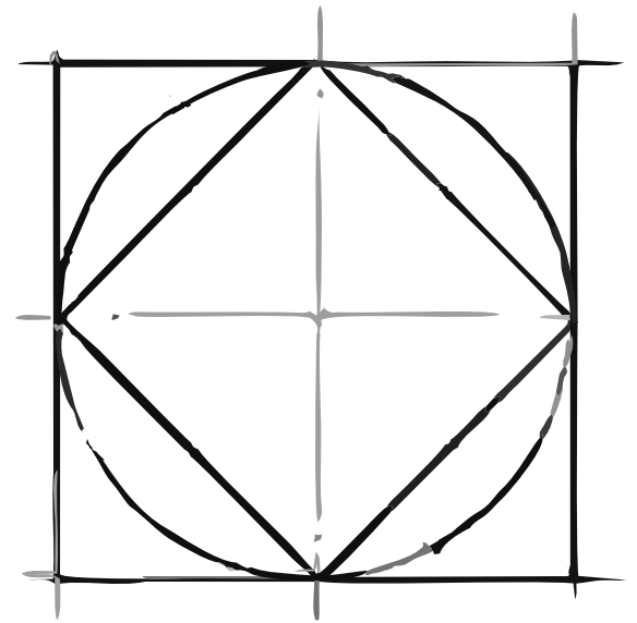
CUADRADO INSCRITO EN CIRCUNFERENCIA 1
