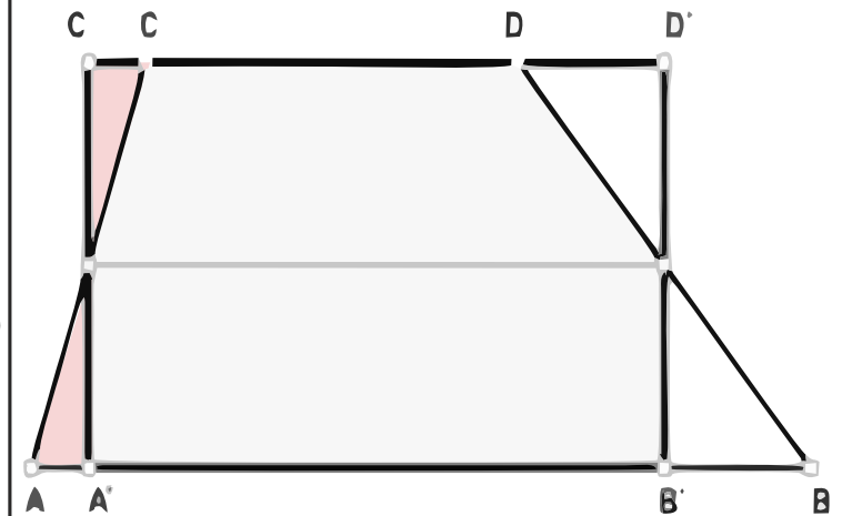
3. TRAPÉCIO SEMEJANTE A UN RECTÁNGULO
