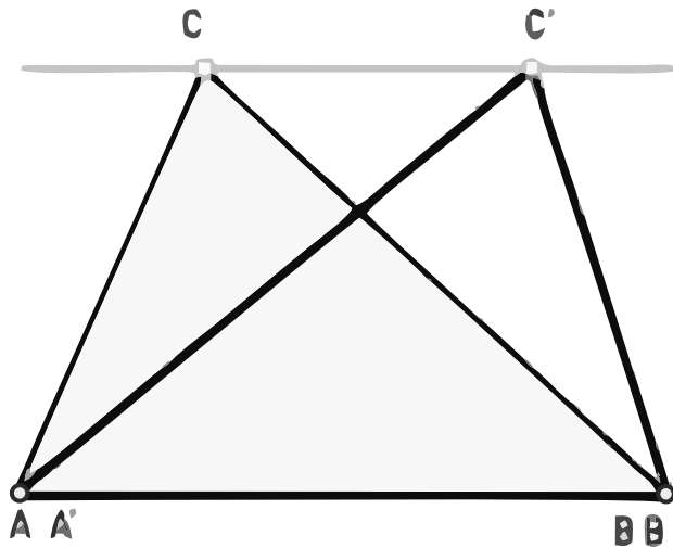
1. EQUIVALENCIA DE TRIÁNGULOS
